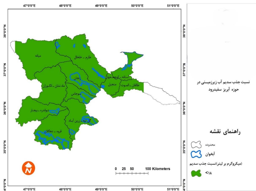
شکل ۴- پهنه‌بندی نسبت جذب سدیم (SAR) آب زیرزمینی در حوزه سفیدرود Fig. 4- Zoning of sodium absorption ratio (SAR) of groundwater in the Sefid-Rud basin
