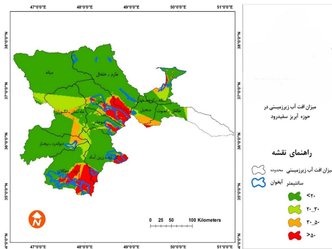
شکل ۵- پهنه‌بندی افت سطح آب زیرزمینی در حوضه سفیدرود Fig. 5- Zoning of groundwater level drop in the Sefid-Rud basin
