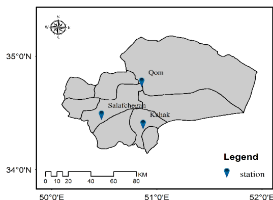
شکل ۱- موقعیت ایستگاه‌های سینوپتیک در استان قم Fig. 1- Location of selected synoptic stations in Qom province
