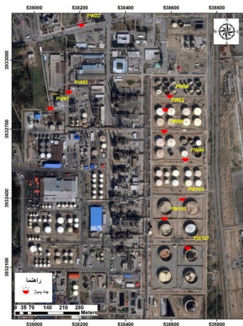
شکل ۲- چاه‌های منتخب برای انجام آزمایش پمپاژ در گستره شهر صنعتی ری (جنوب تهران) Fig. 2- Selected wells for the pumping test in Rey industrial area (south of Tehran)
