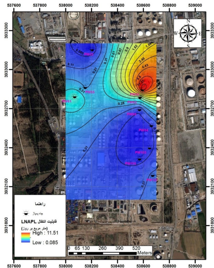
شکل ۵- نقشه هم‌قابلیت انتقال LNAPL به روش کوپر و ژاکوب (Cooper and Jacob, 1946) در گستره مورد مطالعه Fig. 5- Map of LNAPL Iso-Transmissivity using the Cooper and Jacob (1946) method in the study area
