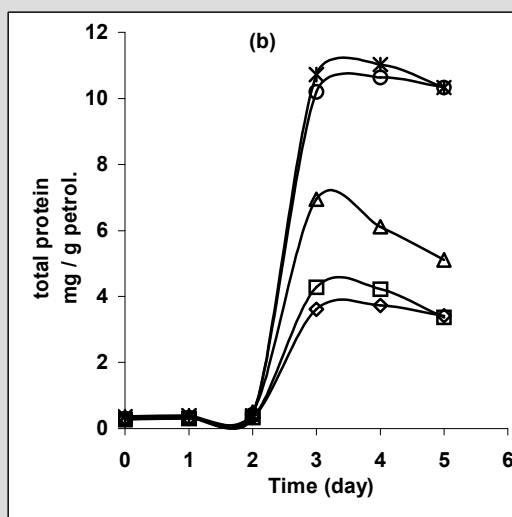
شکل ۲ - بهینه سازی فاکتور میزان P ( \text{Na}_2\text{HPO}_4 ) به ازای هر گرم نفت خام، برای سویه‌های باکتریایی نفت خوار PG01 (a) و PG02 (b) در محیط نفت بعنوان تنها منبع دهنده الکترون. \diamond = 0.006 گرم \text{Na}_2\text{HPO}_4 ، \square = 0.012 گرم \text{Na}_2\text{HPO}_4 ، \triangle = 0.018 گرم \text{Na}_2\text{HPO}_4 ، \circ = 0.024 گرم \text{Na}_2\text{HPO}_4 و * = 0.030 گرم \text{Na}_2\text{HPO}_4
