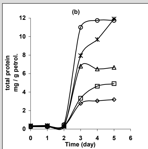
شکل ۱ - بهینه سازی فاکتور میزان N ( \text{NH}_4\text{Cl} ) به ازای هر گرم نفت خام، جهت تجزیه نفت توسط سویه‌های باکتریایی PG01 (a) و PG02 (b) در محیط نفت بعنوان تنها منبع دهنده الکترون. \diamond = 0.049 گرم، \square = 0.097 گرم، \triangle = 0.146 گرم، \circ = 0.195 گرم، * = 0.244 گرم \text{NH}_4\text{Cl}
