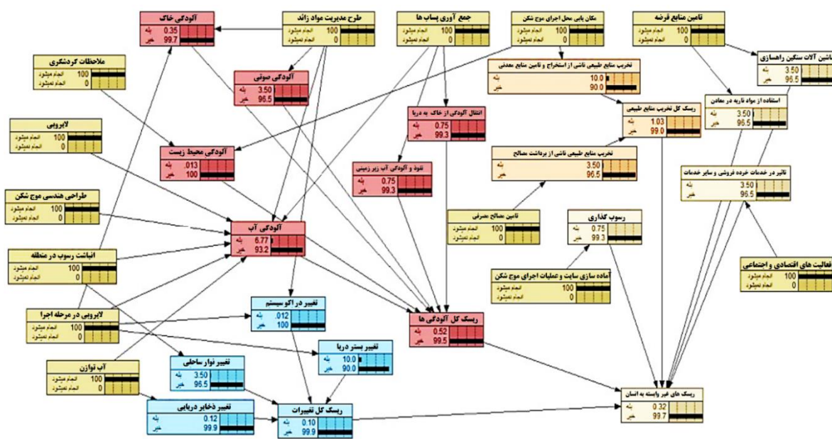
شکل ۶ - مدل احتمال خطرهای غیر وابسته به انسان در موج‌شکن کاسپین Fig. 6- Probability model of non-human-dependent risks in the Caspian Sea breakwater
