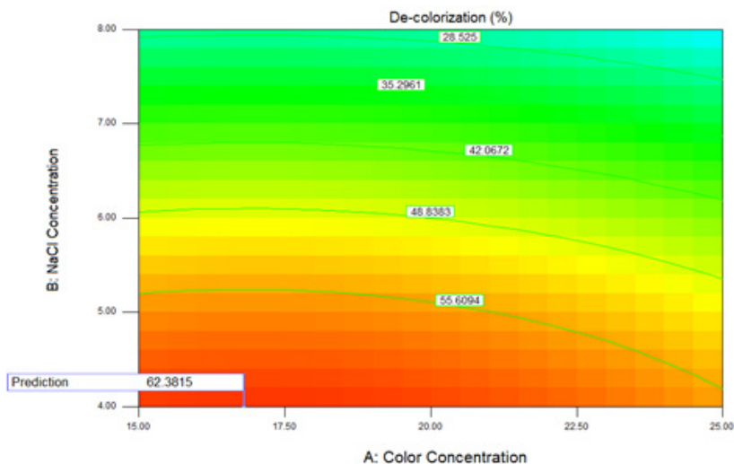
شکل ۵- نتایج بهینه‌سازی میزان تجزیه‌زیستی پساب رنگزا
