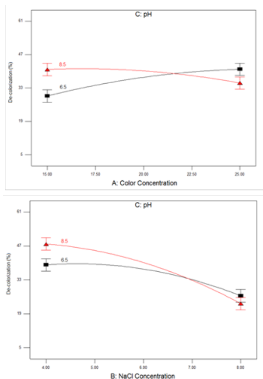
شکل ۴- نمودار اثر های تداخلی متغیرهای دوتایی (الف) غلظت رنگزا و pH (ب) غلظت نمک و pH
