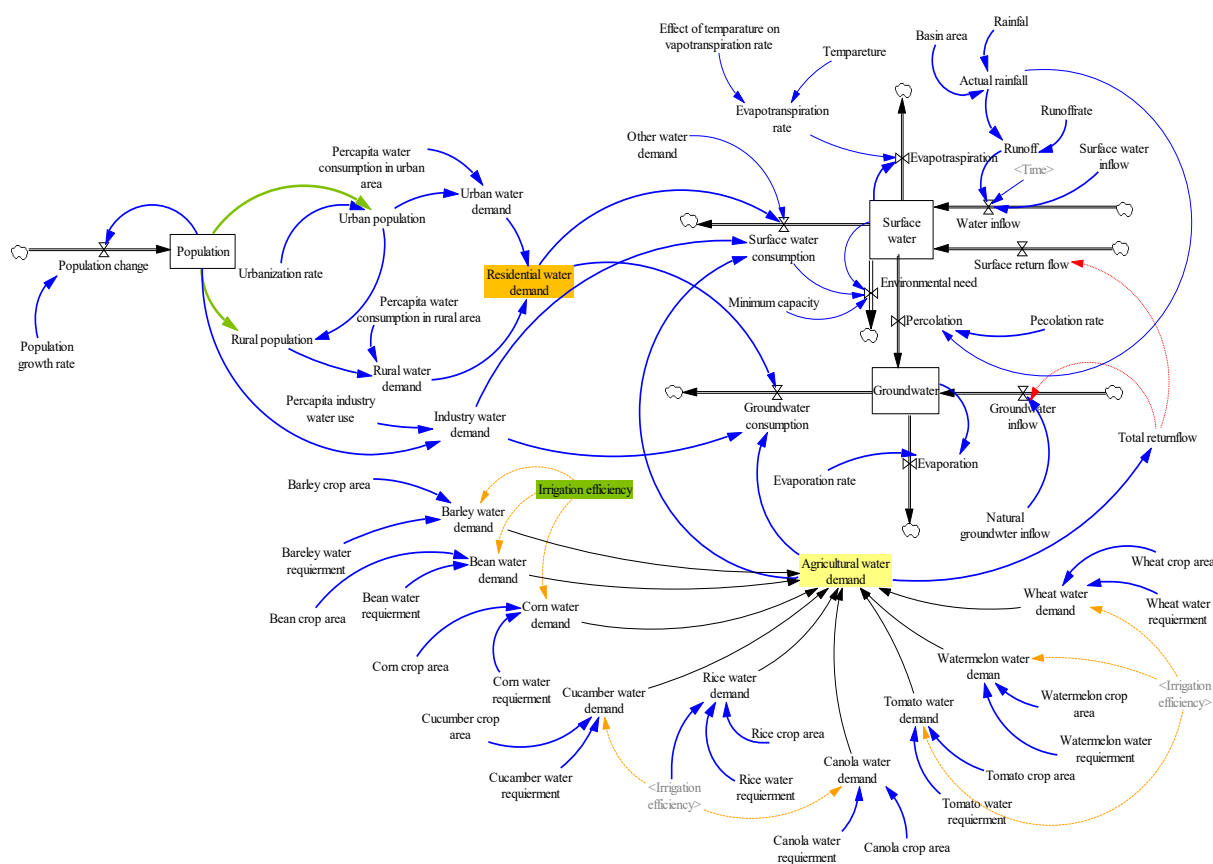
شکل ۲- نمودار ذخیره- جریان سیستم طراحی شده
