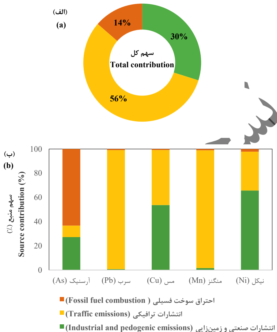
شکل ۵- درصد سهم هر عامل (منبع) بر اساس مدل APCS/MLR (الف) و درصد سهم هر عامل (منبع) در انتشار عناصر آرسنیک، سرب، مس، منگنز و نیکل (ب) در خاک شهری همدان
