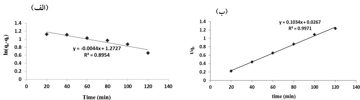
شکل ۶- نمودارهای سینتیک (الف) شبه درجه اول و (ب) شبه درجه دوم مربوط به جذب آفلاتوکسین B 1
