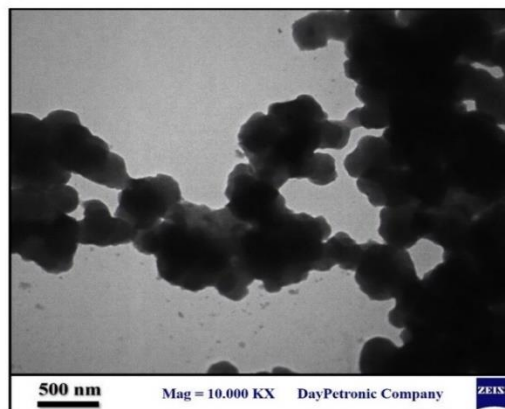
شکل ۲- تصویر TEM مربوط به \text{Fe}_3\text{O}_4\text{-Au@MIP} Fig.2- TEM image of \text{Fe}_3\text{O}_4\text{-Au@MIP}
