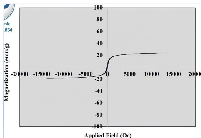
شکل ۴- نمودار VSM مربوط به MMIP
