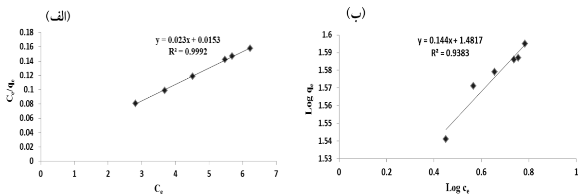
شکل ۷- نمودار ایزوترم‌های (الف) لانگمویر و (ب) فروندلیچ مربوط به جذب آفلاتوکسین B 1
