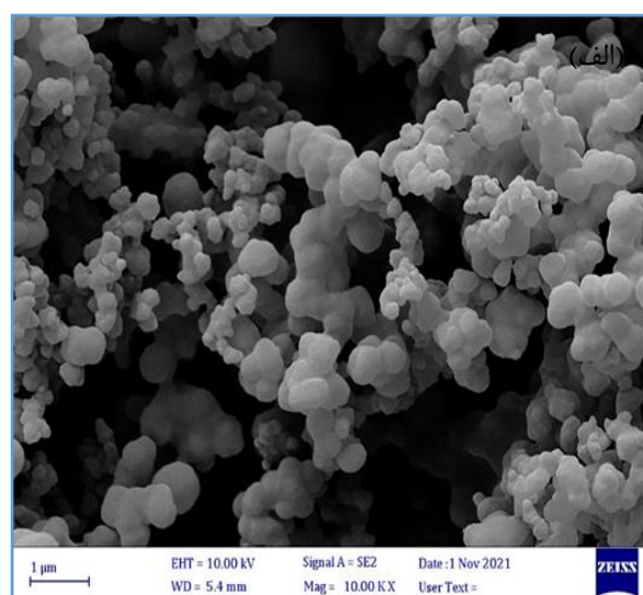
شکل ۱- تصاویر FESEM مربوط به \text{Fe}_3\text{O}_4\text{-Au@MIP} (الف) و پلیمر قالب مولکولی به همراه سم آفلاتوکسین (ب)
