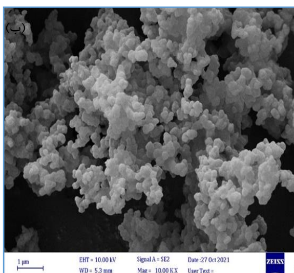
شکل ۱- تصاویر FESEM مربوط به \text{Fe}_3\text{O}_4\text{-Au@MIP} (الف) و پلیمر قالب مولکولی به همراه سم آفلاتوکسین (ب)
