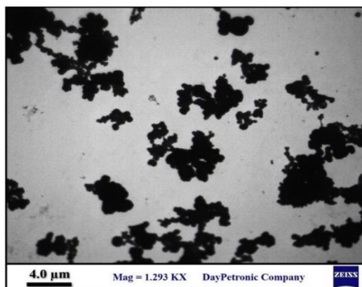
شکل ۲- تصویر TEM مربوط به \text{Fe}_3\text{O}_4\text{-Au@MIP} Fig.2- TEM image of \text{Fe}_3\text{O}_4\text{-Au@MIP}
