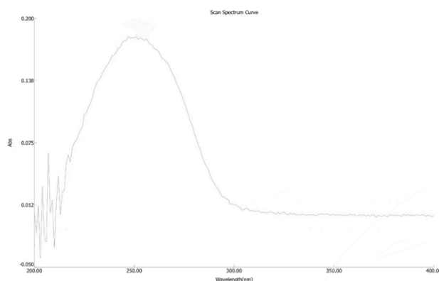
شکل ۹- طیف جذبی آفلاتوکسین B 1
