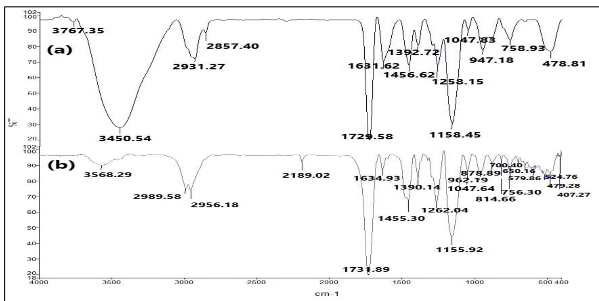
شکل ۳- طیف FTIR مربوط به \text{Fe}_3\text{O}_4\text{-Au@MIP} شسته نشده (a) ، و \text{Fe}_3\text{O}_4\text{-Au@MIP} شسته شده (b)
