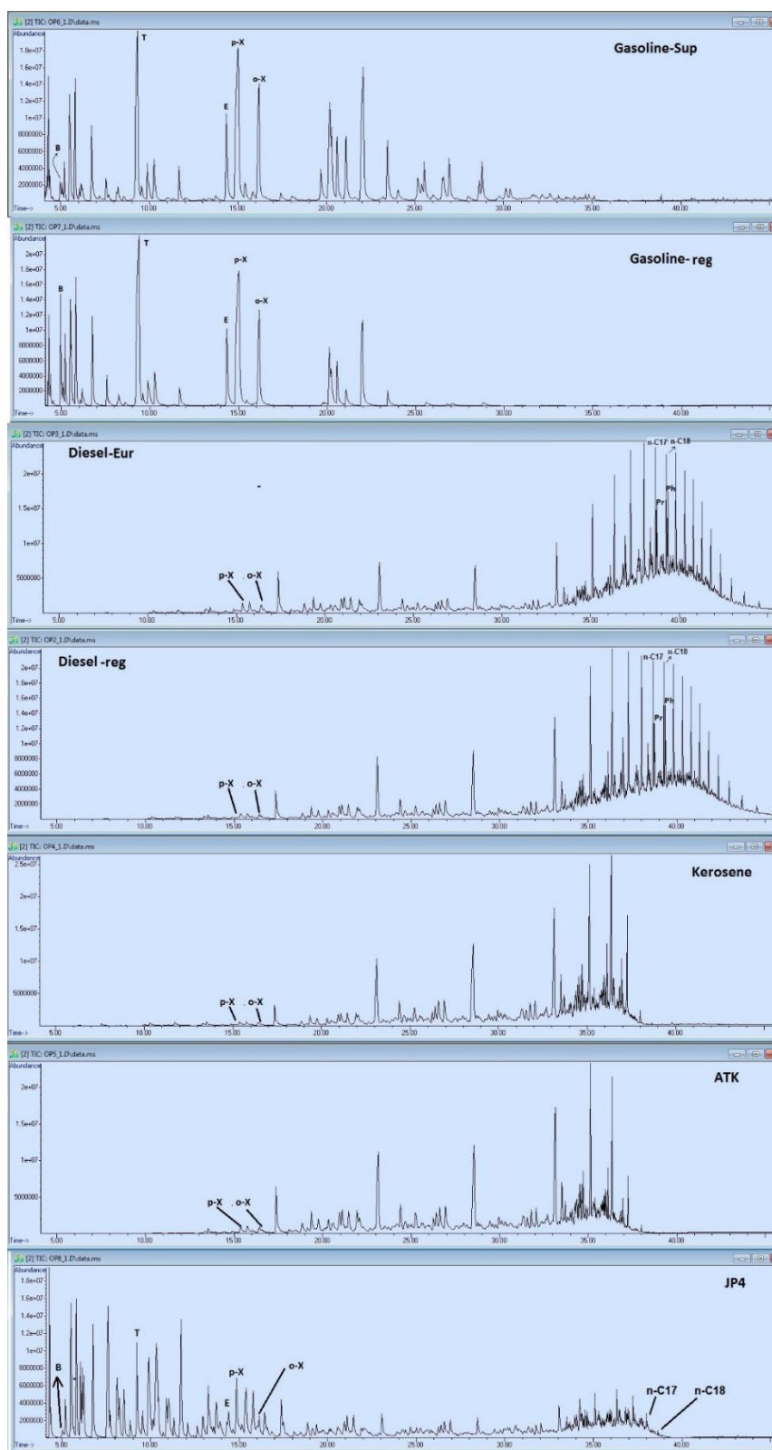
شکل ۳- کروماتوگرام‌های GC-MS دو نوع بنزین و دیزل در مخازن بالای سطح زمین (B: بنزن، T: تولوئن، E: اتیل بنزن، p-X: پارا-زایلن، o-X: اورتو-زایلن، n-17: هپتادکان، n-18: اکتادکان، Pr: پریستین، Ph: فایتین، reg: معمولی، Eur: یورو).
