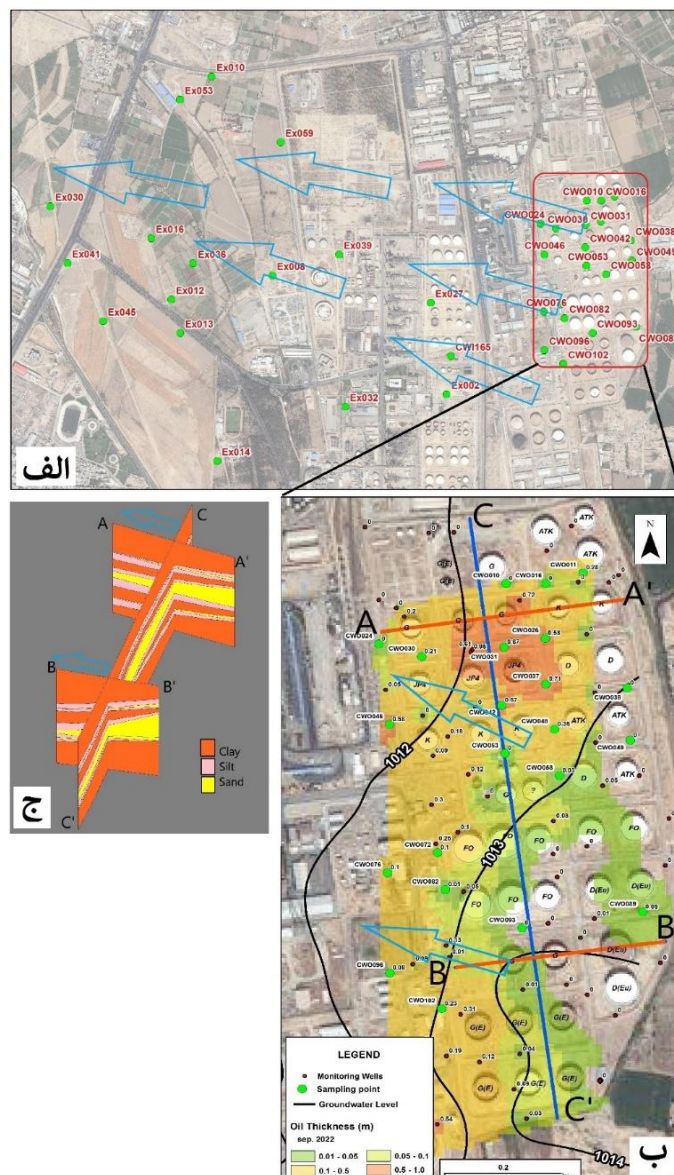
شکل ۱- محدوده مطالعاتی و موقعیت نقاط نمونه برداری جهت: الف) ارزیابی میرایی طبیعی آبخوان، ب) تفکیک منشأ (چهار گوش قرمز رنگ) و ج) نمودار فانس مقاطع عرضی (A, B, C) رسوبات تشکیل دهنده آبخوان. جهت جریان آب زیرزمینی (فلش آبی)، خطوط هم‌پتانسیل سطح آب زیرزمینی (خطوط سیاه)، ضخامت آلودگی در شهریور ۱۴۰۱ (نوار رنگی) و موقعیت مخزن‌های بالای سطح زمین که حاوی ATK، بنزین سوپر (G_E)، بنزین (G)، نفت سفید (K)، سوخت جت (JP4)، دیزل (D)، دیزل یورو (D_Eu) و نفت کوره (FO) می باشند Fig 1- Study area and location of sampling points for: a) evaluation of natural attenuation of the aquifer, b) source differentiation (red quadrants), and c) fence diagrams of cross sections (A, B, C) of the aquifer-forming sediments. Groundwater flow direction (blue arrows), groundwater level equipotential lines (black lines), pollution thickness in September 2022 (colored bands), and location of above-ground tanks containing ATK, premium gasoline (G_E), gasoline (G), kerosene (K), jet fuel (JP4), diesel (D), Euro diesel (D_Eu), and fuel oil (FO) are shown.
