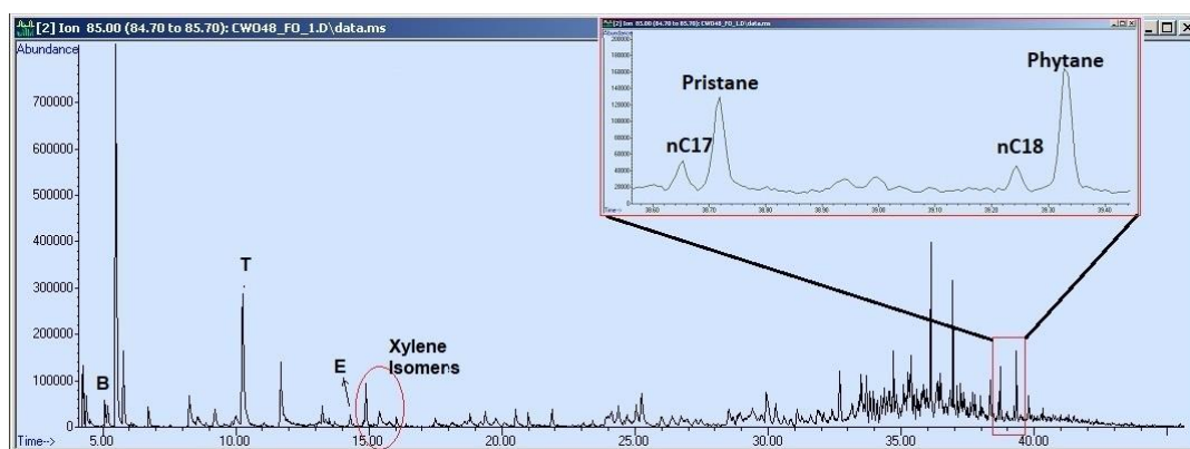
شکل ۴- کروماتوگرام GC-MS نفت شناور در نمونه CWO48 در منطقه A که اختلاط بنزین و دیزل را نشان می‌دهد Fig. 4 - GC-MS chromatogram of floating oil in sample CWO48 in area A, indicating a mixture of gasoline and diesel.
