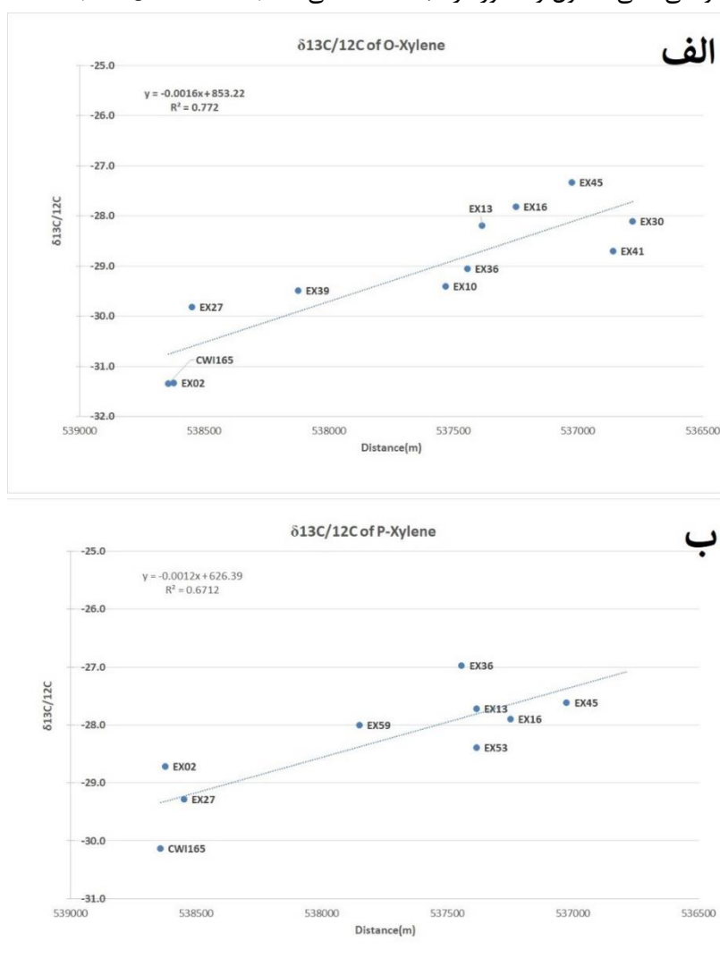
شکل ۱۰- افزایش نسبت ایزوتوپی \delta^{13}C/^{12}C در ترکیب الف) o-Xylene (۴ پرمیل در ۱۷۰۰ متر)، ب) p-Xylene (۴ پرمیل در ۱۵۰۰ متر)،
