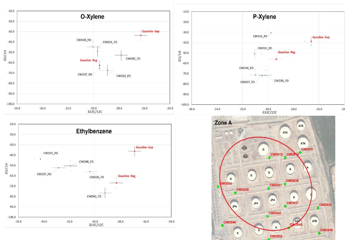
شکل ۶- نمودار دو بعدی از مقادیر \delta^{13}\text{C} در مقابل مقادیر \delta^2\text{H} اتیل بنزن، o -زایلین و p -زایلین در نمونه‌های مواد نفتی شناور که نوع بنزین معمولی به جای سوپر (مخلوط با دیزل در منطقه A را نشان می‌دهد)
