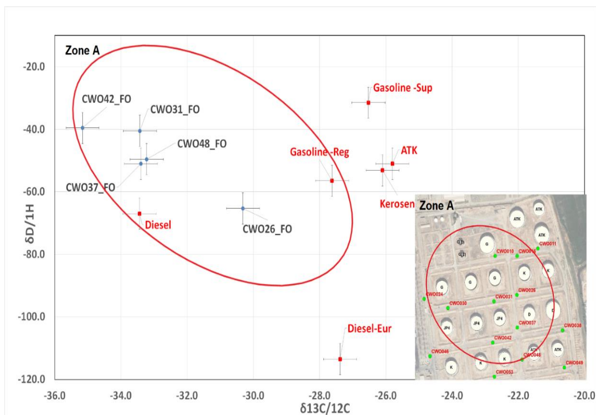
شکل ۵- نمودار دو بعدی مقادیر \delta^{13}\text{C} در برابر \delta^2\text{H} تولوئن در نمونه‌های نفت شناور Fig. 5 - Two-dimensional plot of \delta^{13}\text{C} values versus \delta^2\text{H} values for toluene in floating oil samples
