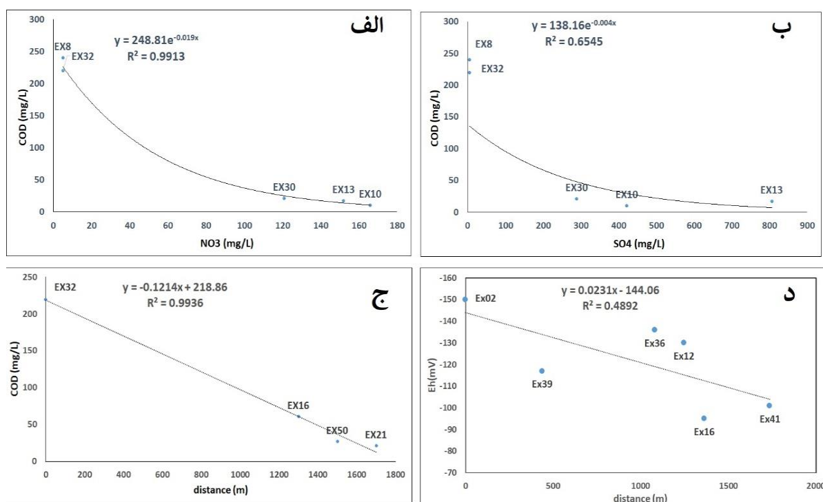
شکل ۹- تغییرات نیترات (الف) و سولفات (ب) در مقابل COD به عنوان غلظت آلاینده های آلی، (ج) غلظت COD و (د) ارزش Eh در مقابل فاصله در یک خط جریان آب زیرزمینی
