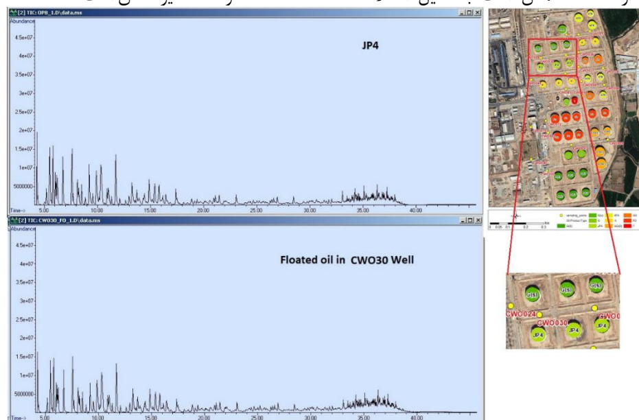
شکل ۸- تطابق کامل کروماتوگرام JP4 با نمونه روغن شناور از چاه CWO30، واقع در نزدیکی مخزن بالادست حاوی JP4، که منشأ
