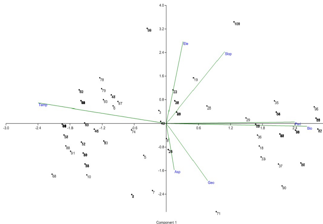
شکل ۶ - نمودار تجزیه به مولفه‌های اصلی: O. microcarpa (1-40)، O. elwendica (44-69)، O. bilabiata (87-89)، O. subsericea (41-43)، O. bulbotricha (90-95)، O. sabalanica (96-100)، O. sericea (73-75)، O. cornuta (86-86)، O. chlorotricha (70-72)، 43 Fig. 6- PCA diagram of species: O. microcarpa (1-40), O. elwendica (44-69), O. bilabiata (87-89), O. subsericea (41-43), O. chlorotricha (70-72), O. cornuta (86-86), O. sericea (73-75), O. sabalanica (96-100), O. bulbotricha (90-95)
