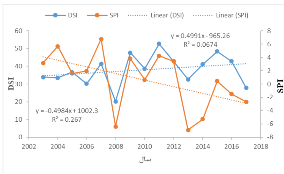
شکل ۹- رابطه همبستگی بین شاخص‌های DSI و SPI در استان سمنان Fig. 9- Correlation relationship between SPI and DSI indices in Semnan Province
