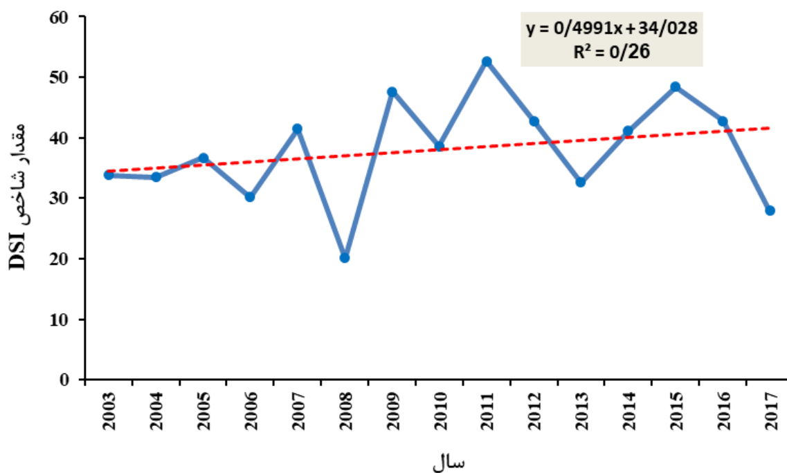
شکل ۷- روند شاخص طوفان گرد و غبار (DSI) در طول سال‌های مورد مطالعه در استان سمنان
