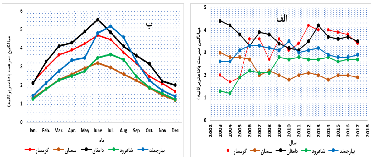
شکل ۴- نمودار تغییرات بلندمدت سرعت باد غالب سالانه (الف) و ماهانه (ب) ایستگاه‌های سینوپتیک استان سمنان Fig. 4- Chart of long-term changes in annual (a) and monthly (b) prevailing wind speed of synoptic stations in Semnan Province
