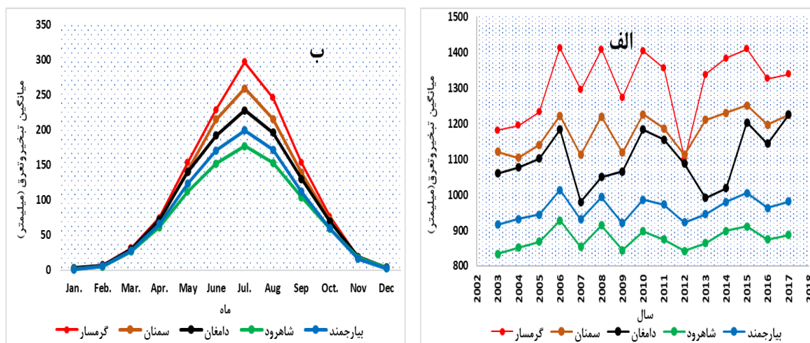
شکل ۵- نمودار تغییرات بلندمدت تبخیر و تعرق پتانسیل سالانه (الف) و ماهانه (ب) ایستگاه‌های سینوپتیک استان سمنان Fig. 5- Chart of long-term changes of annual (a) and monthly (b) evapotranspiration potential of synoptic stations of Semnan Province
