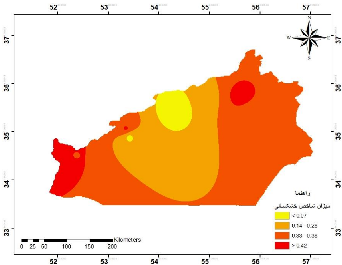
شکل ۶- نقشه پراکندگی خشکسالی استان سمنان در بازه زمانی ۲۰۱۷-۲۰۰۳ Fig. 6- Drought distribution map of Semnan Province in the period of 2003-2017
