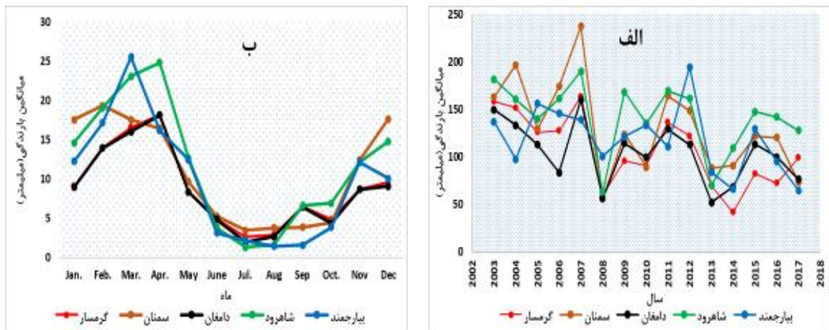
شکل ۲- نمودار تغییرات بلندمدت بارش سالانه (الف) و ماهانه (ب) ایستگاه‌های سینوپتیک استان سمنان Fig. 2- Chart of long-term changes of annual (a) and monthly (b) precipitation of synoptic stations of Semnan Province
