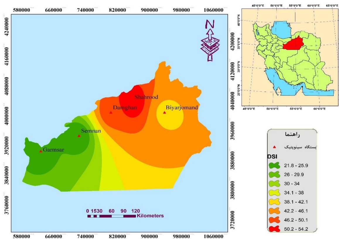
در مناطق مختلف استان در دوره آماری ۱۵ ساله (۲۰۰۳-۲۰۱۷) DSI شکل ۸- پهنه‌بندی وضعیت تغییرات شاخص
