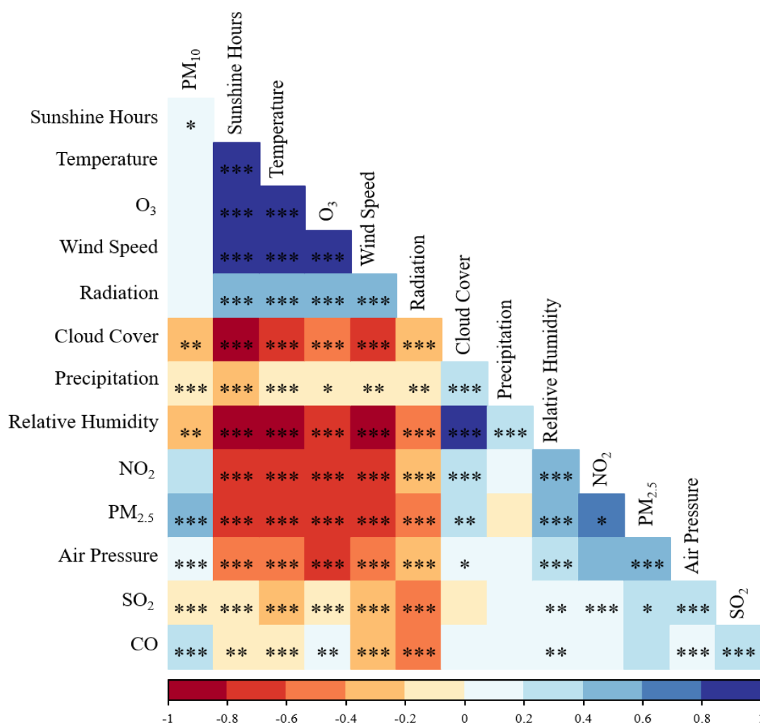
شکل ۶- ضریب همبستگی پیرسون میان عناصر هواشناسی و آلاینده‌های جوی معیار در مقیاس زمانی ماهانه در شهر تبریز (۲۰۲۱-۲۰۰۴) Fig. 6- Pearson's correlation coefficient between meteorological elements and criteria air pollutants in the monthly time scale in Tabriz during 2004- 2021
