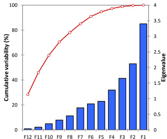
شکل ۱۲- نمودار صخره‌ای جزیره گرمایی شهرستان اصفهان با روش PCA
