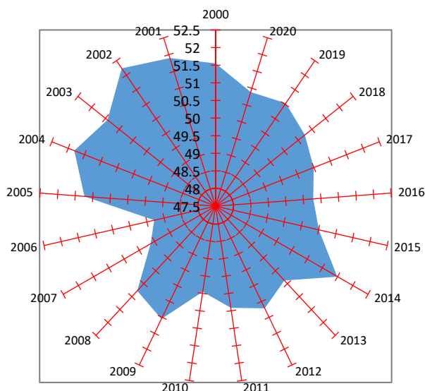
شکل ۷- کیلوگرام از توزیع پراکنش جزیره حرارتی در ماه آگوست Fig. 7- Kilogram of heat island distribution in August
