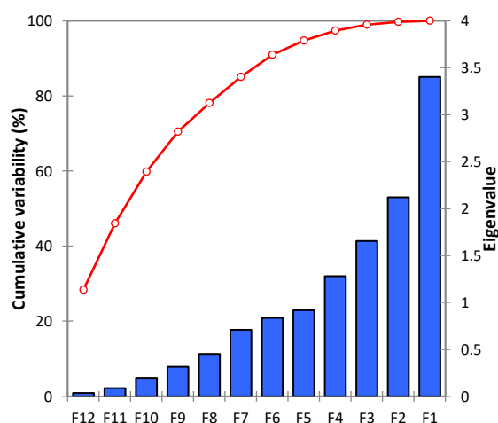
شکل ۱۲- نمودار صخره‌ای جزیره گرمایی شهرستان اصفهان با روش PCA Fig. 12- Scree plot of heat island in Isfahan County with PCA method
