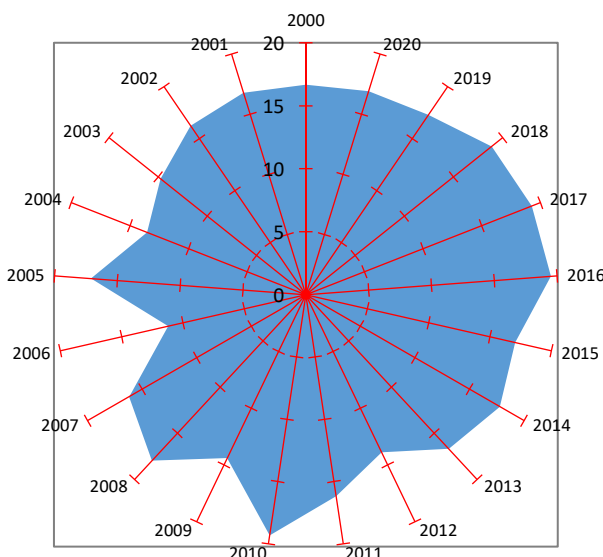
شکل ۸- کیلوگرام از توزیع پراکنش جزیره حرارتی در ماه دسامبر Fig. 8- Kilogram of heat island distribution in December
