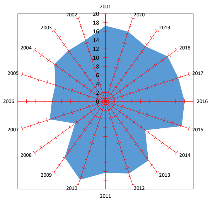
شکل ۶- کلموگرام از توزیع پراکنش جزیره حرارتی در ماه ژانویه Fig. 6- Kilogram of heat island distribution in January
