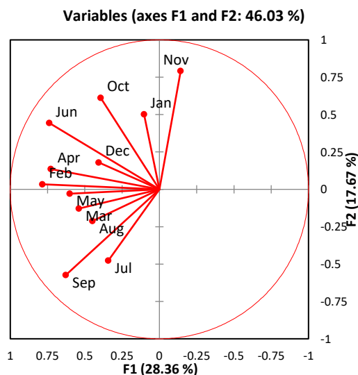
شکل ۱۳- نمودار پراکنش جزیره‌حرارتی شهرستان اصفهان با روش PCA Fig. 13- Scatter plot of heat island in Isfahan County with PCA method
