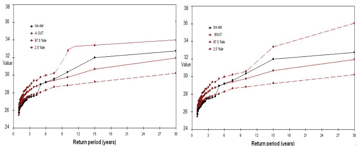
شکل ۲- نمودار دوره برگشت چرخه‌های معنی دار میانگین دمای سالانه با مدل HadCM 3 در سناریوی A 2 (چپ) و B 2 (راست) در ایستگاه ایزه
