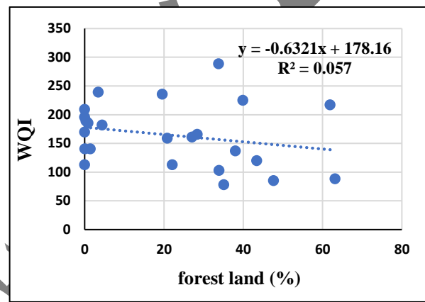
الف. ارتباط درصد کاربری جنگل و WQI
