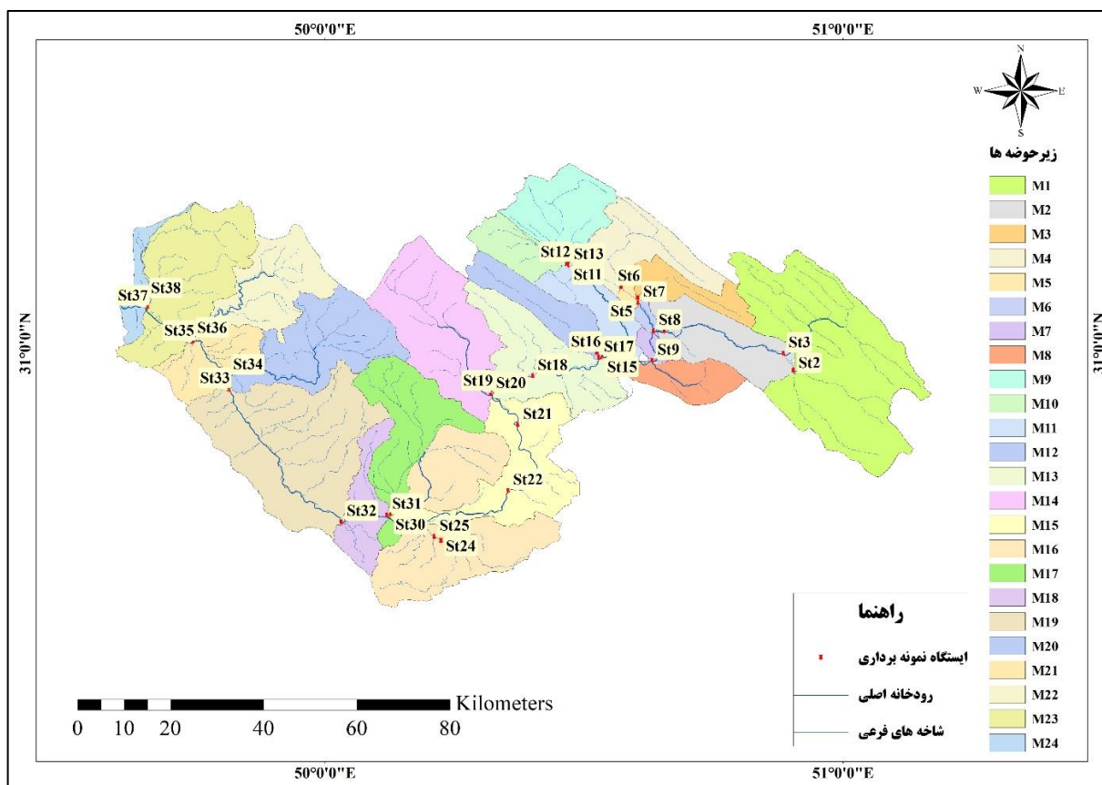
شکل ۱- نقشه موقعیت زیرحوضه‌ها، شبکه رودخانه و ایستگاه‌های نمونه برداری در زیرحوضه آبخیز رودخانه مارون Fig. 1- Location map of sub-basins, river network and sampling stations in Maroon River sub-basin
