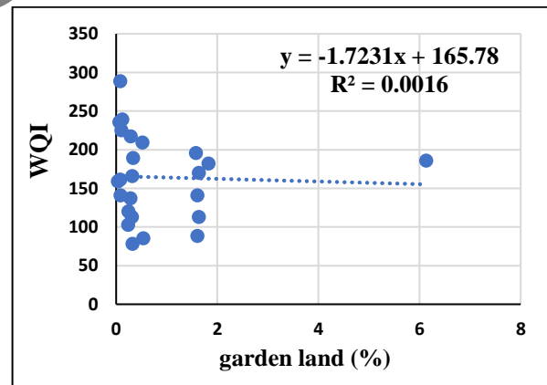
ج. ارتباط درصد کاربری باغ و WQI
