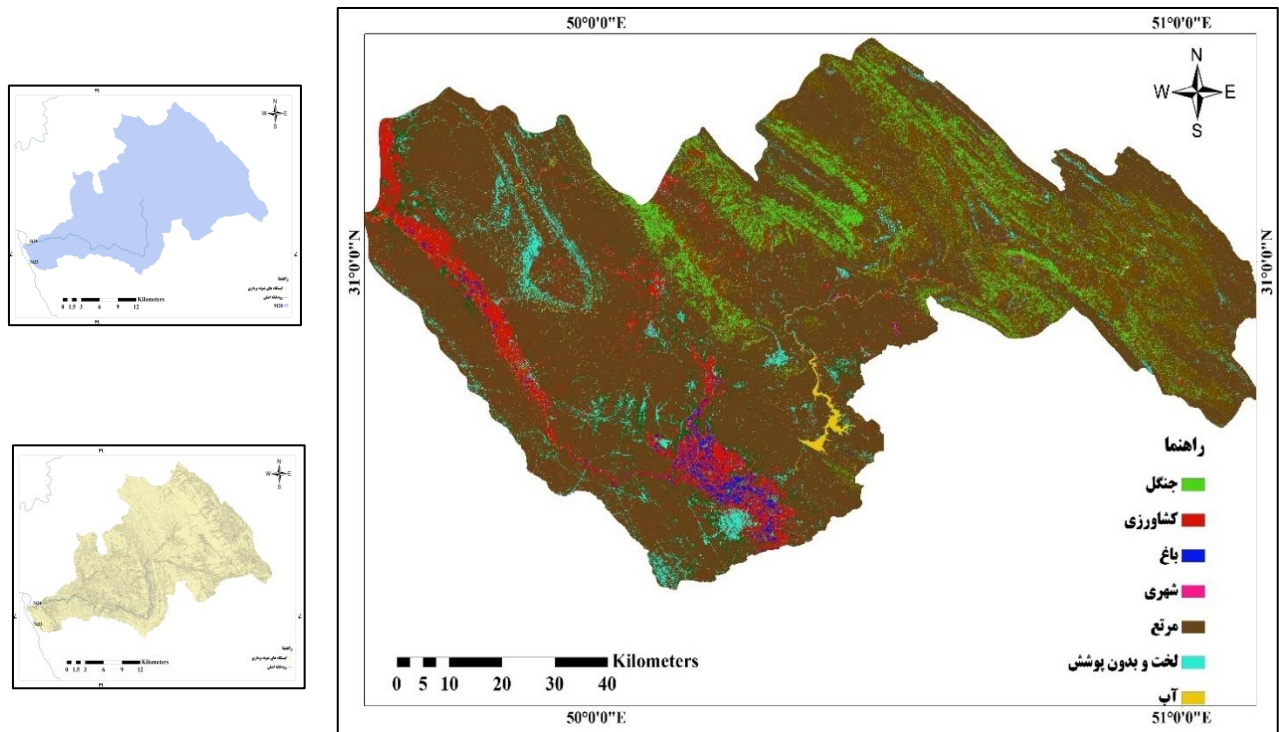
شکل ۳- نقشه الگوهای کاربری اراضی در زیرحوضه آبخیز رودخانه مارون Fig. 3- Map of land use patterns in the Maroon River sub-basin
