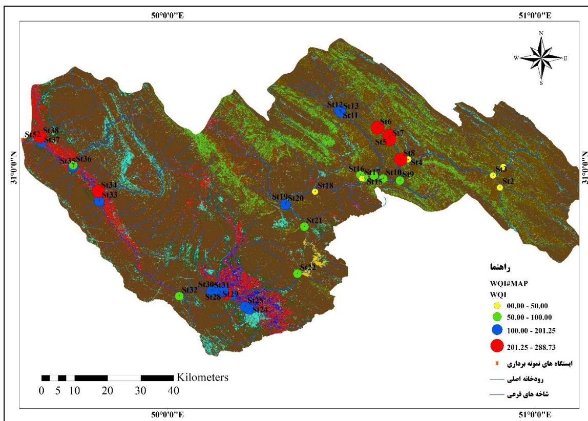
شکل ۷- همبستگی فضایی بین الگوهای کاربری اراضی و شاخص کیفیت آب زیرحوضه رودخانه مارون Fig. 7- Spatial correlation between land use patterns and water quality index of Maroon River sub-basin
