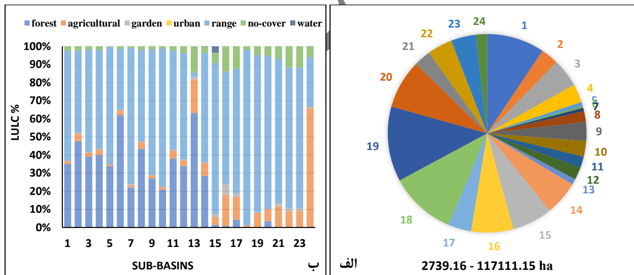
شکل ۴- الف) مساحت کل زیرحوضه‌ها و ب) درصد الگوهای کاربری‌های مختلف اراضی در زیرحوضه‌ها Fig. 3- a) total area of sub-basins, and b) percentage of different land use patterns in sub-basins
