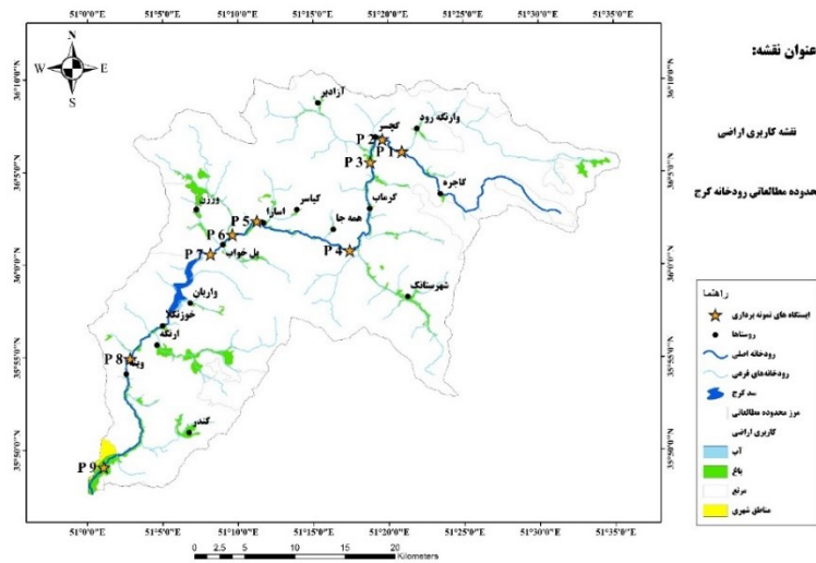
شکل ۲- نقشه ی نقاط نمونه برداری و کاربری اراضی رودخانه ی کرچ Fig. 2- Map of sampling points and land use of Karaj River
