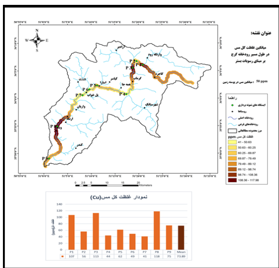
شکل ۳- نقشه های تغییرات غلظت عناصر سنگین در طول مسیر رودخانه Fig. 3- The maps of heavy metals' concentration changes along the river
