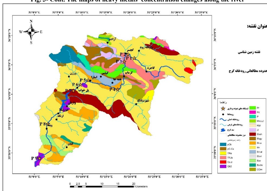
شکل ۴- نقشه ی زمین شناسی رودخانه ی کرج Fig. 4- Geological map of Karaj River
