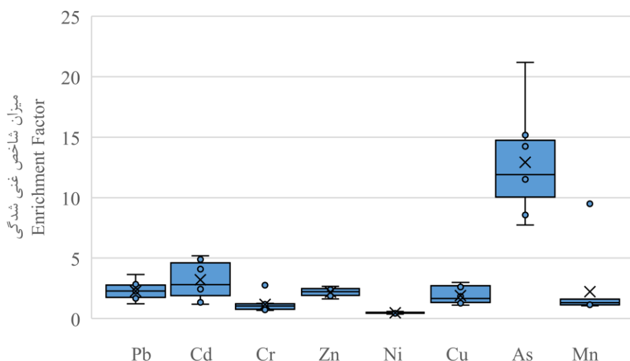
شکل ۶- نمودار جعبه ای شاخص غنی شدگی عناصر سنگین رسوبات رودخانه ی کرج بر مبنای آلومینیوم
