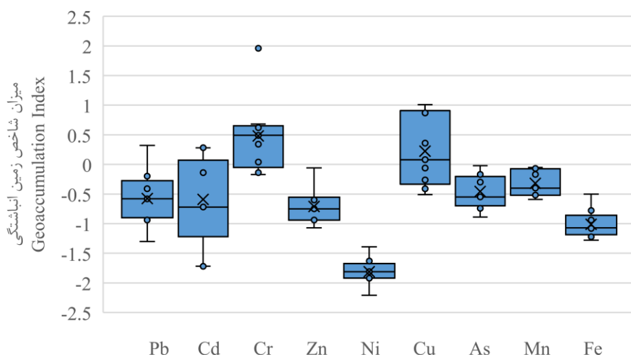
شکل ۵- نمودار جعبه ای شاخص زمین انباشتی عناصر سنگین رسوبات رودخانه ی کرج Fig. 4- Boxplot diagram of heavy metals' Geoaccumulation Index in Karaj River sediments
